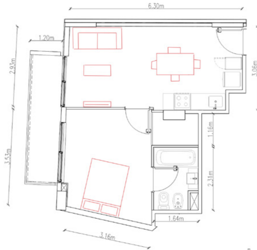
UF 101 2 AMB 36,8 m 2 + BALCÓN
