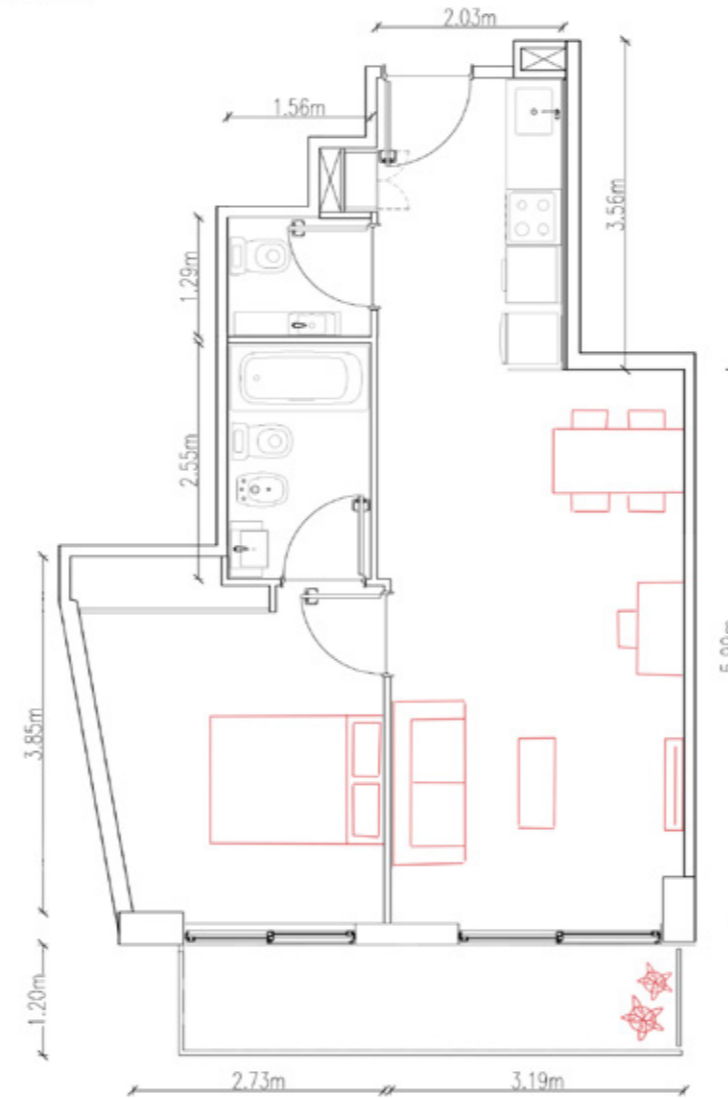
UF 102 - 202 2 AMB 46,2 m 2 + BALCON 6,5 m 2
